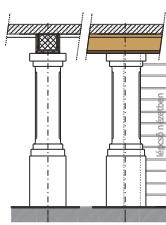
NÉZET_02
