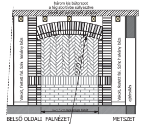
BELSŐ OLDALI FALNÉZET METSZET
