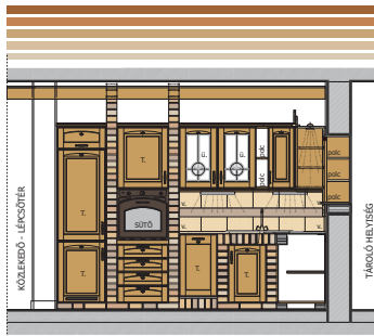
BELSŐÉPÍTÉSZET - KONYHABÚTOR TERVE
