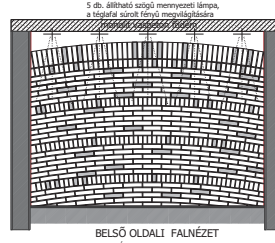
BELSŐ OLDALI FALNÉZET TEGLARÖKÖLÁTÁS FAL
