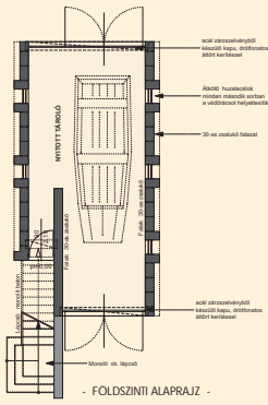
- FÖLDSZINTI ALAPRAJZ -
