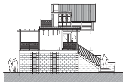
- ÉSZAKKELETI HOMLOKZAT -
