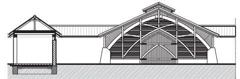
Szénatároló - Dél nyugati homlokzat
