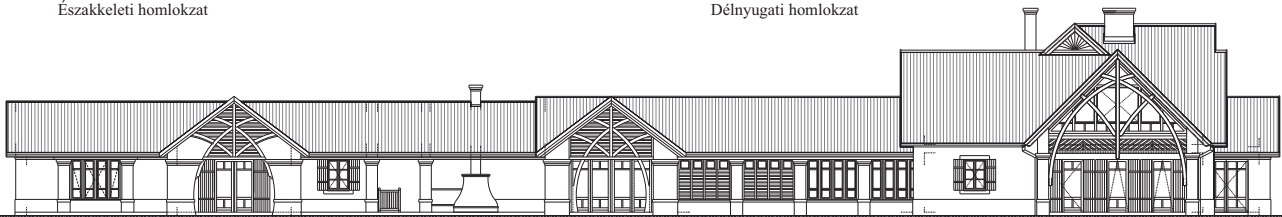
Délkeleti homlokzat
