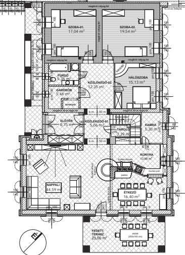
- Földszinti Alaprajz -
