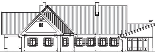
Északkeleti homlokzat
